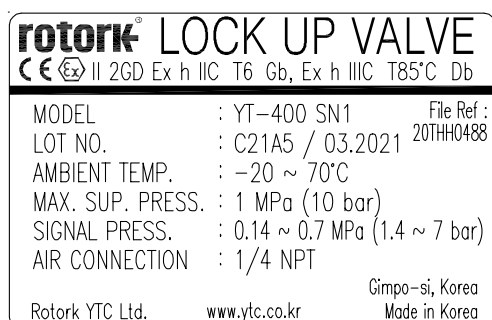
Fig. L-1: YT-400 (ATEX)
