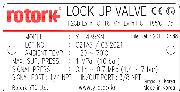
Fig. L-7: YT-435 (ATEX)
