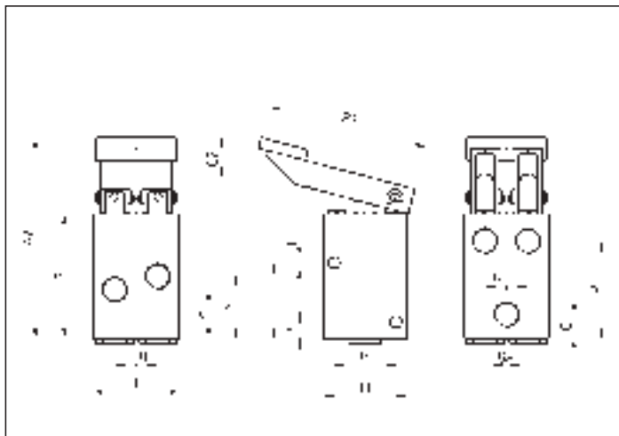
5/2 TAPPER
