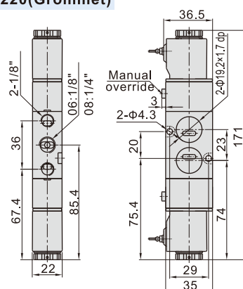
4M220(Grommet)
