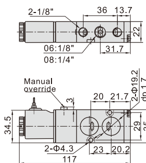
4M220(Grommet)
