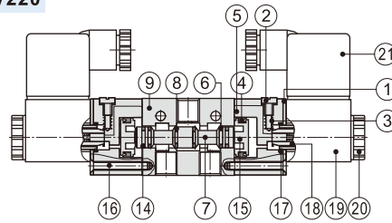
3V220
