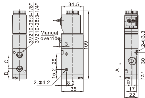
3V210(Grommet)
