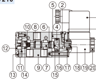
3V210
