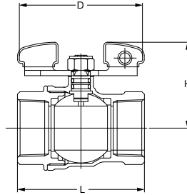
Dimensions of AKSAW, CSAW
