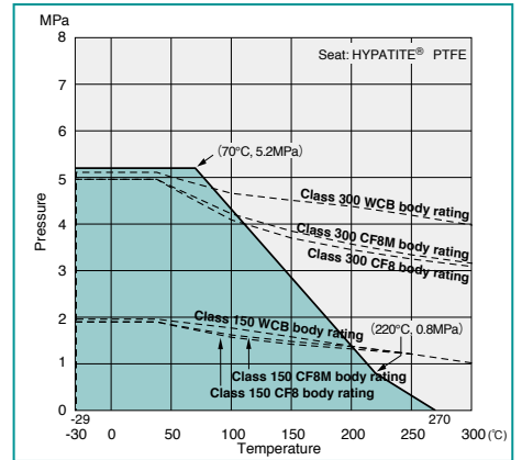
150/300UTDZ(M)/SCTD : NPS 3, 4
