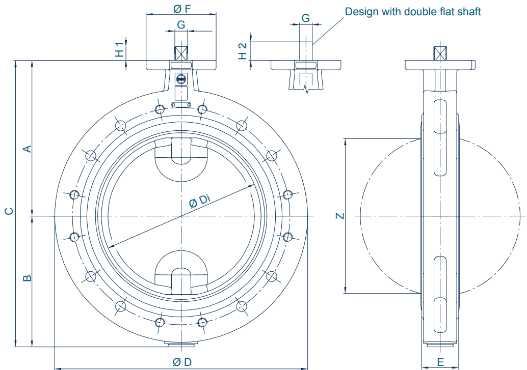
Z 612-A with bare shaft end acc. to EN ISO 5211
